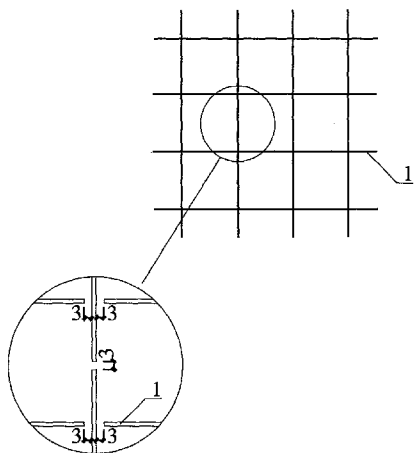
图 5.4.4 防静电水磨石地面铜(或不锈钢)分格条接头处理
